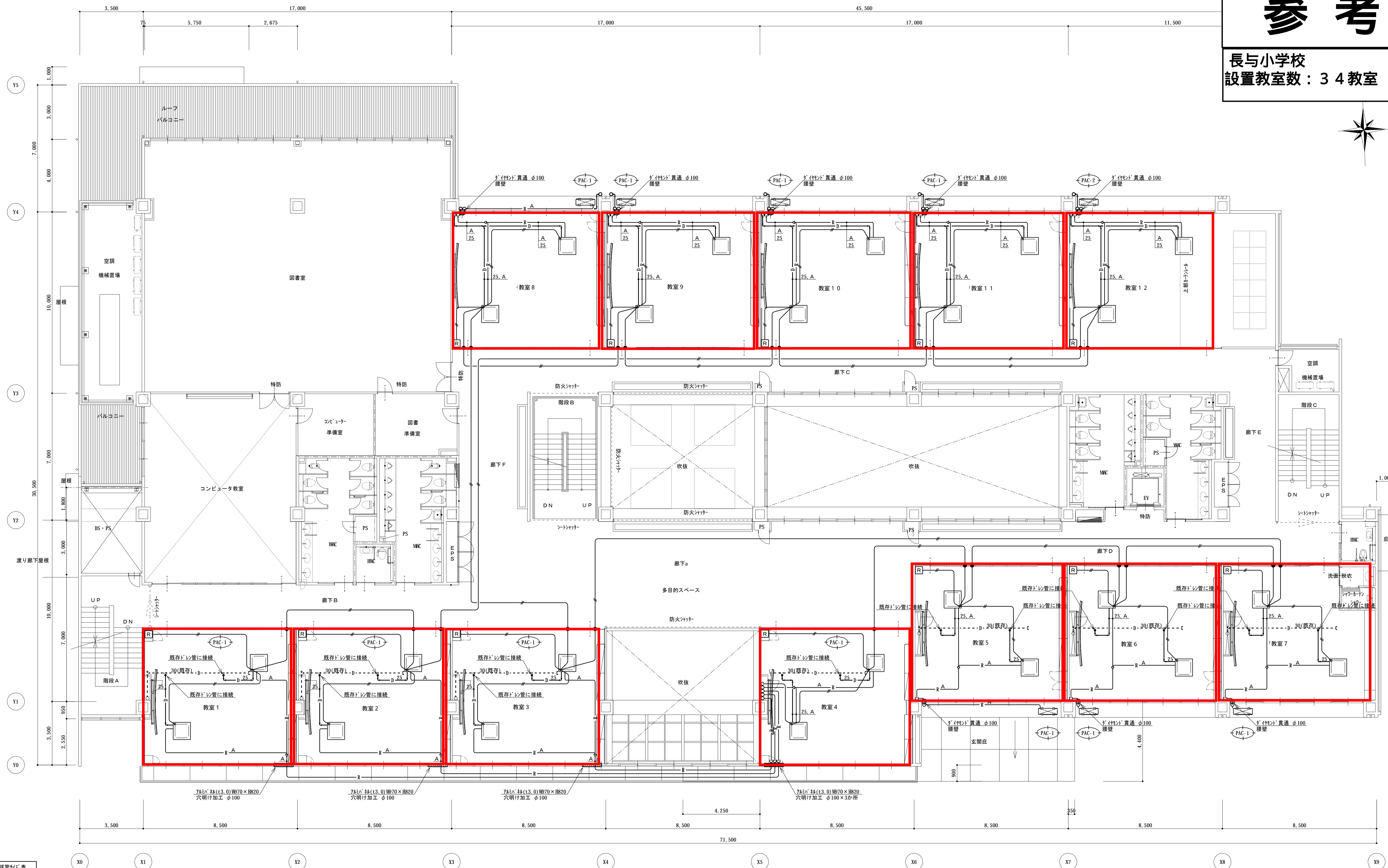
空調設備 2階平面図 A1=1/100 ※●は、防火区画貫通処理・ダクト貫通 φ50を示す。
