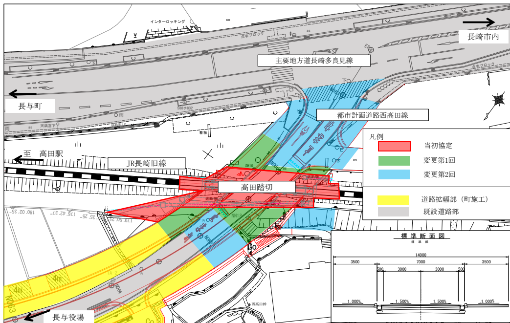
図-1 平面図
