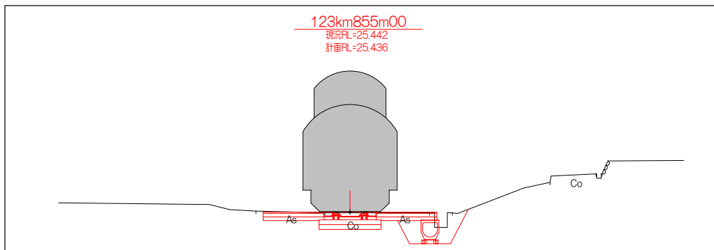
図-2 線路横断面
