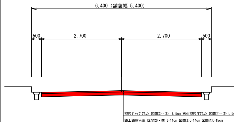
標準断面図
