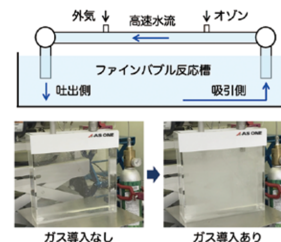
図2 空気ファインバブルで洗浄 (白濁は微細なオゾンの泡が浮遊している状態)
