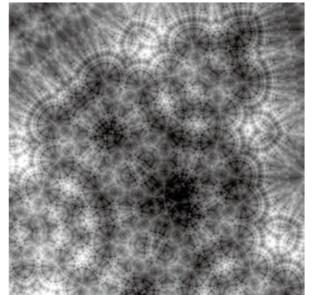
図2：紙を折り続ける造形シミュレーション
