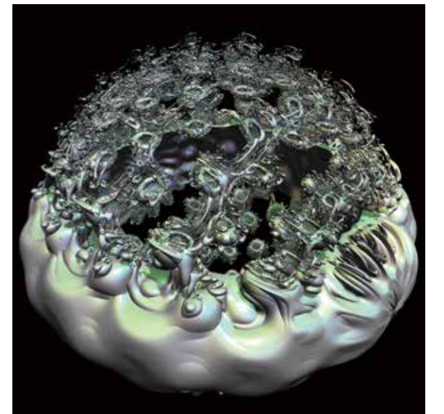
図1：疑似三元数によるフラクタル
