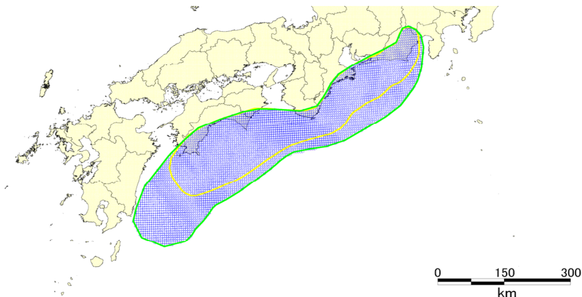
四連動モデル（東海・東南海・南海・日向灘）（Mw9.0）断層配置図
