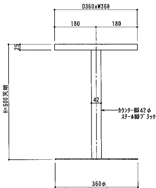
カウンター:姿図
