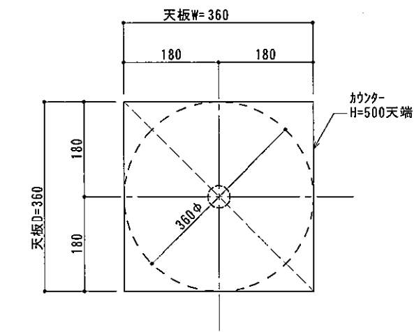
カウンター:平面図
