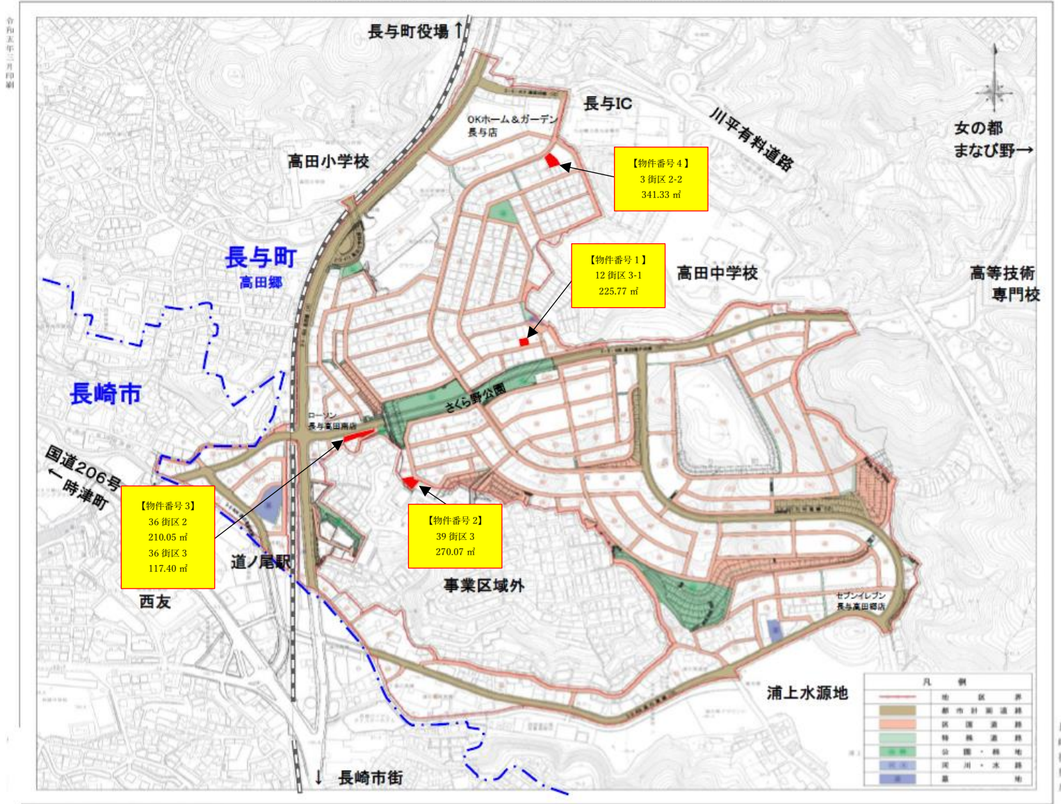
長崎都市計画事業高田南土地区画整理事業計画図
